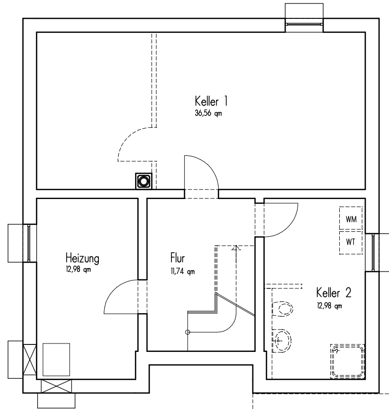
Kellergeschoss
